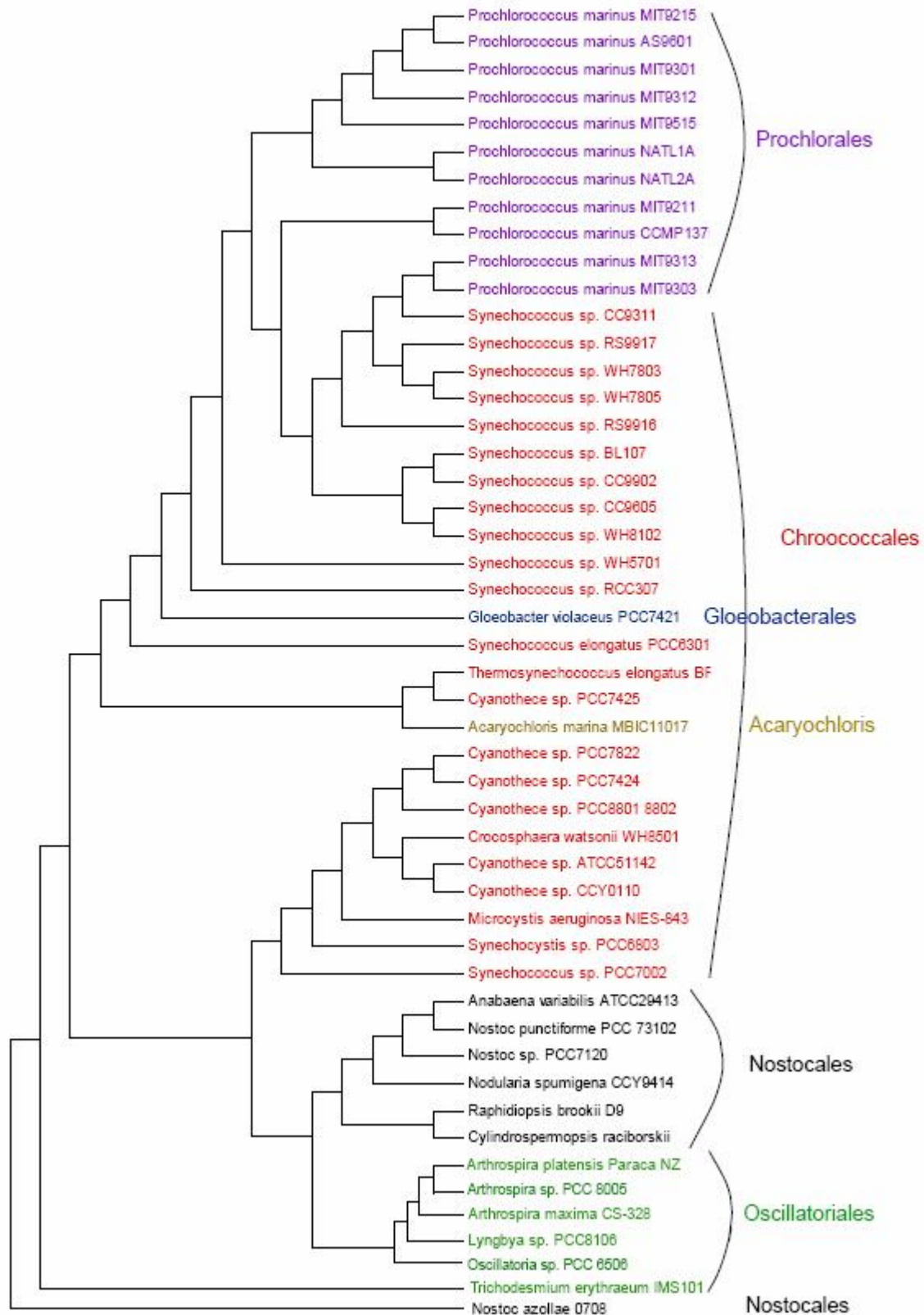
Рисунок 5. Дерево NtcA-фактора у цианобактерий. Цветами выделены таксономические порядки. Видно, что близость фактора хорошо согласована с близостью видов.
